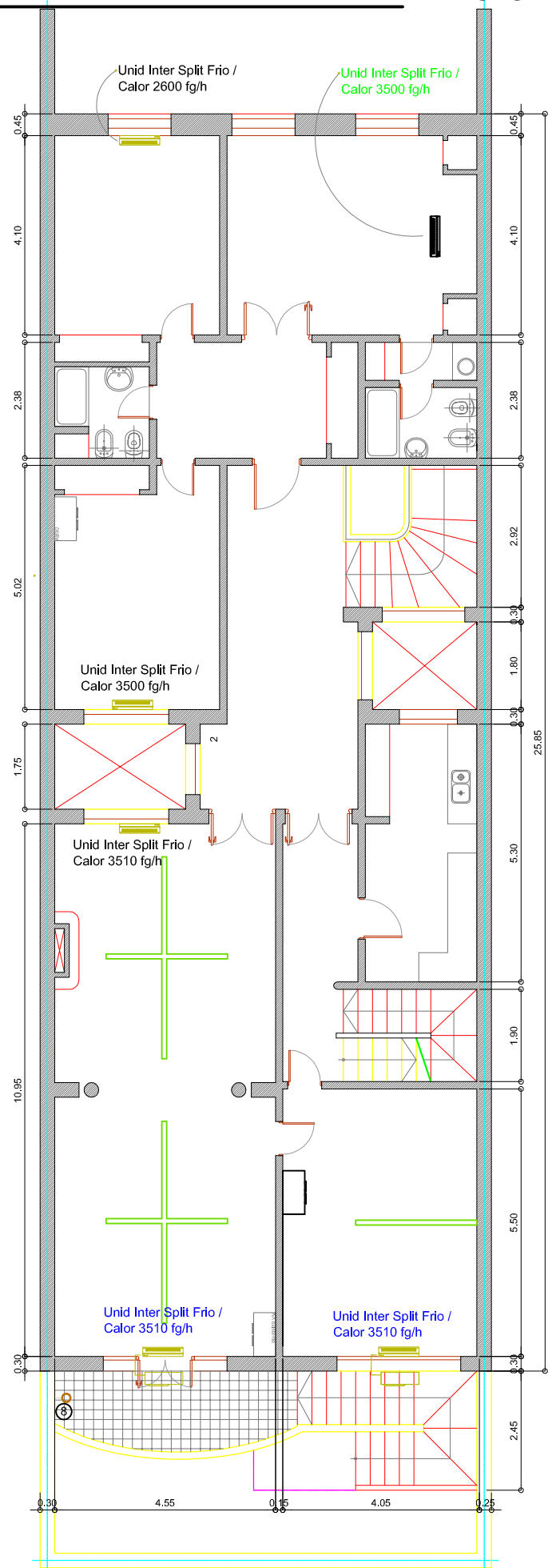
PLANTA ALTA
